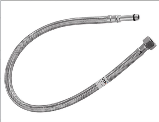
Single Base Hose Length: 45, 60 cm Size: 1/2" x 1/2", 3/8" x 3/8" Dia: 12 mm Material: Wire S.S/ Aluminum شیلنگ تک پایه طول: ۴۵، ۶۰ سانتی متر سایز: ۱/۲ x ۱/۲ اینچ، ۳/۸ x ۳/۸ اینچ ضخامت: ۱۲ میلی متر متریال: استیل یا آلومینیوم
